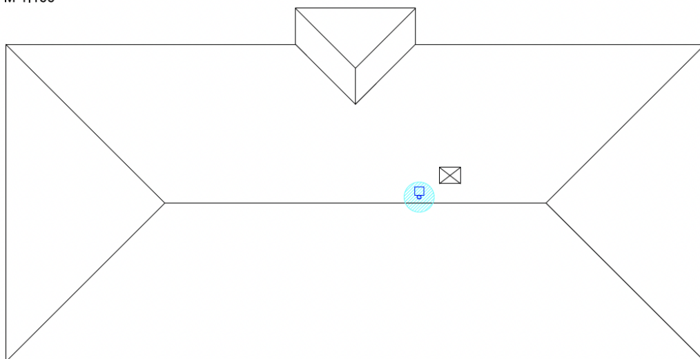
PŮDORYS STŘECHY M 1:100
